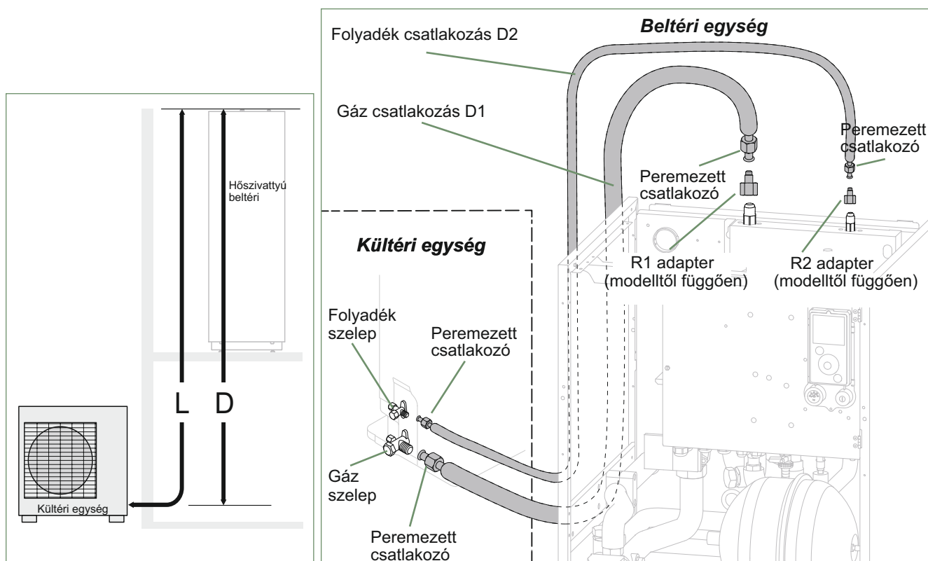
19. ábra - Kálorikus csatlakozások
