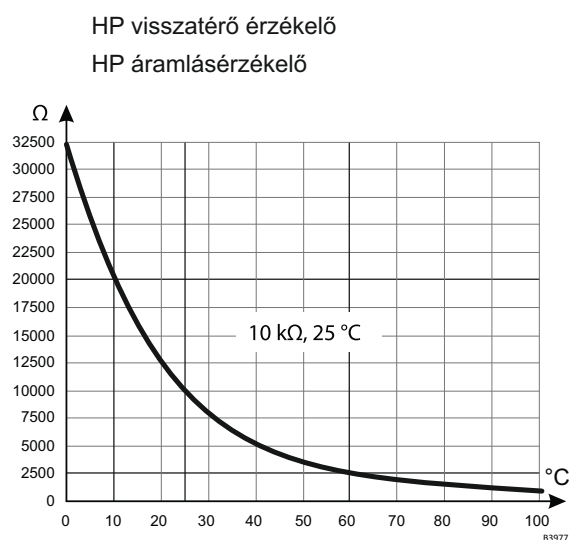
6. ábra - Ohmikus érzékelő értékek (belső egység)
