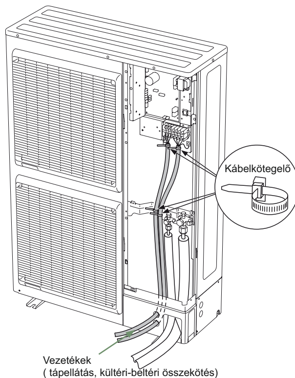
39. ábra - Bekötés véglegesítése 3 fázisú kültéri egységnél
