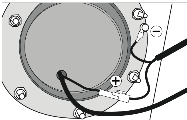
57. ábra - ACI ellenőrzés
