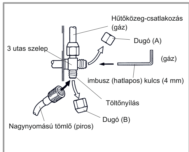
22. ábra - A tömlő csatlakoztatása a gázszelephoz
