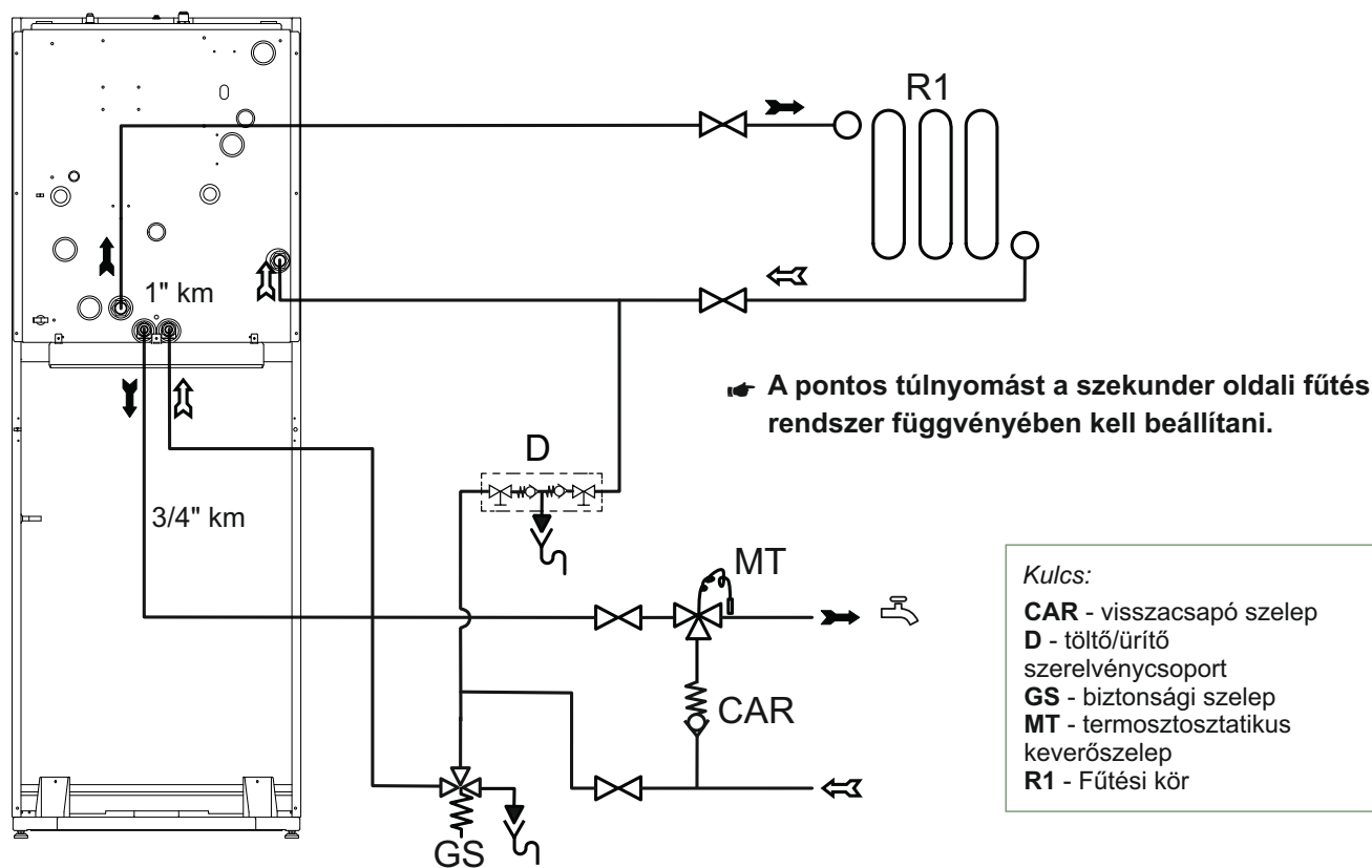
25. ábra - Egyszerűsített vízőldali bekötés
