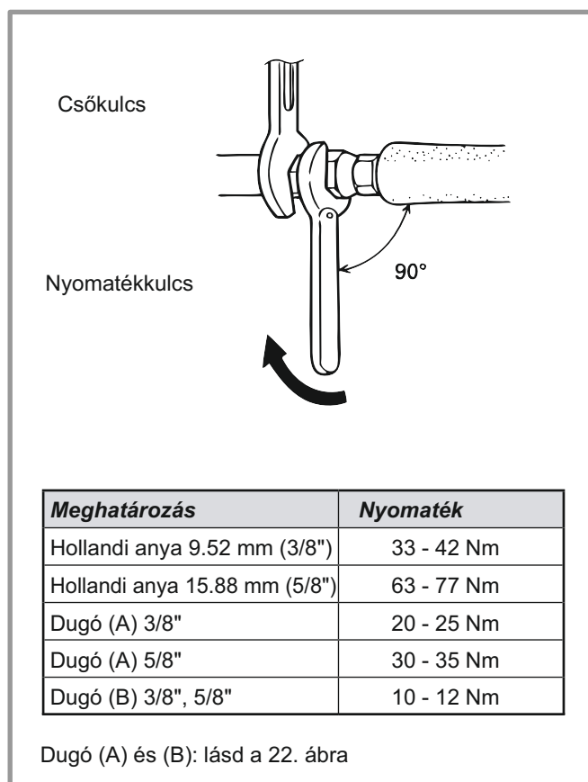
20. ábra - meghúzási nyomatékok
