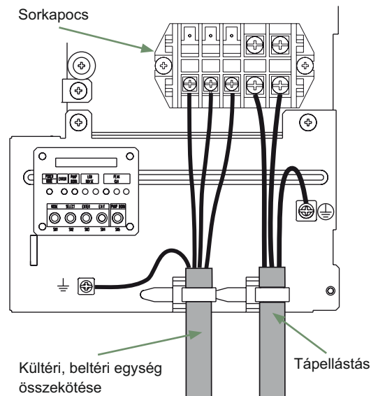
35. ábra - Kültéri egység villamos bekötése
