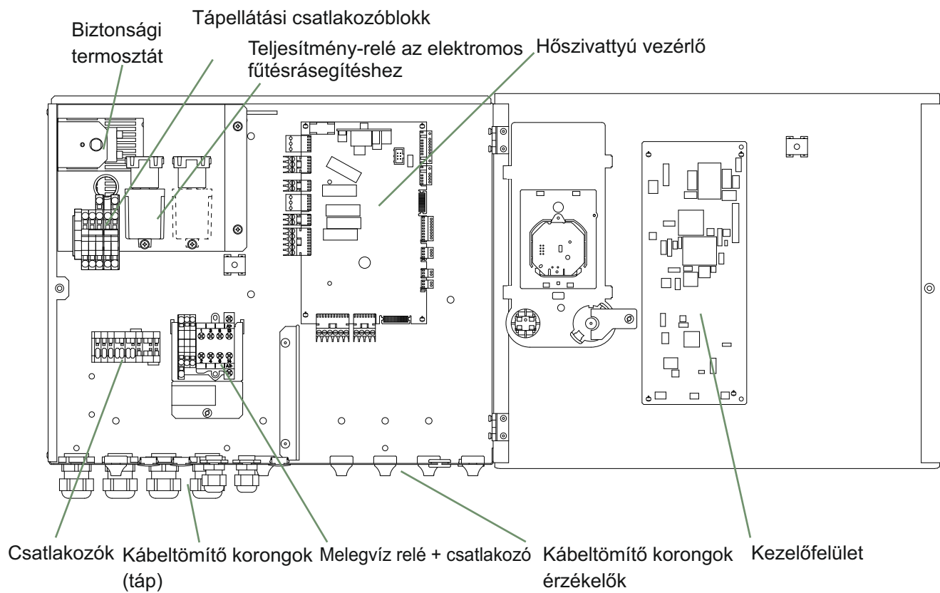
42. ábra - Az egy fázisú beltéri egység elektromos vezérlődoboz
