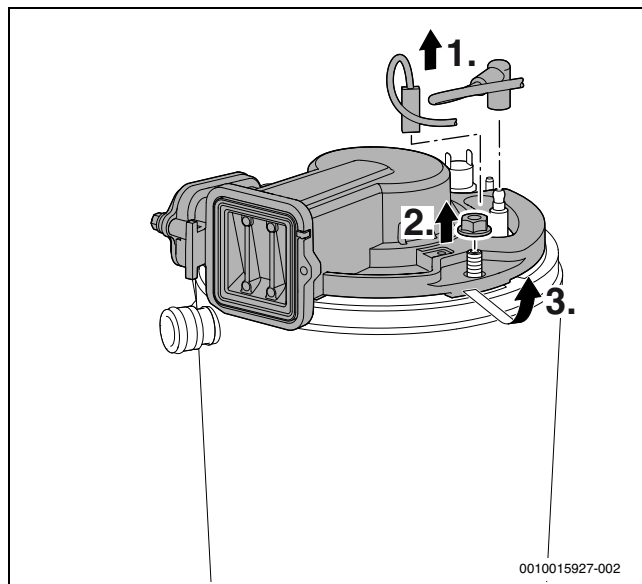
51. ábra Az égőfedél leoldása
