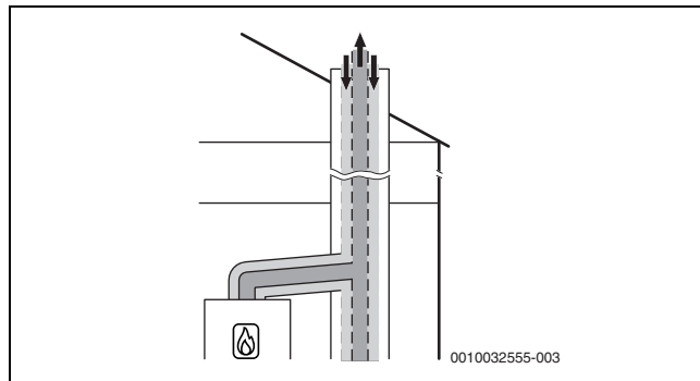
9. ábra A C 43x szerinti koncentrikus levegő-/füstgázelvezetés a felállítási helyiségben
