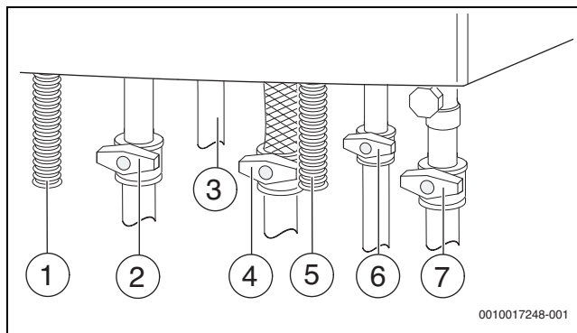
34. ábra Gáz- és vízdali csatlakozások (külön rendelhető tartozékok)
