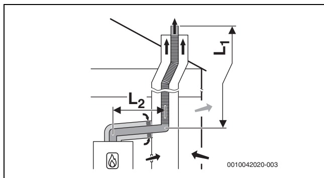
16. ábra B_{53p} szerinti flexibilis füstgázvezetés aknában, környezeti levegőtől függő levegőellátással a felállítási helyiségben lévő koncentrikus összekötő vezetékén keresztül; hátsó szellőzőnyílás az aknában
