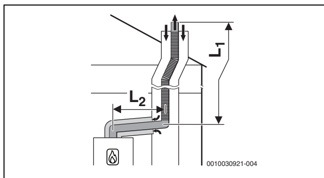
14. ábra Flexibilis égéstermék-elvezetés a C 63x szerint aknában és koncentrikus levegő-/égéstermék-elvezetés a felállítási helyiségben
