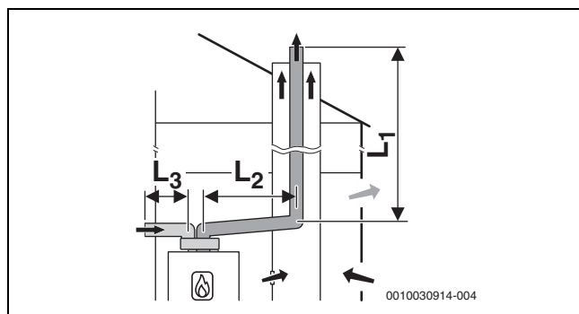
10. ábra Merev fűtgázvezetés a C 53 szerint az aknában és különálló, egyfalú levegőellátó-/fűtgáz-vezetékek a felállítási helyiségben
