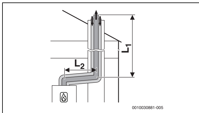
7. ábra Koncentrikus levegő-/ füstgázelvezetés a C 33x szerint az aknában
