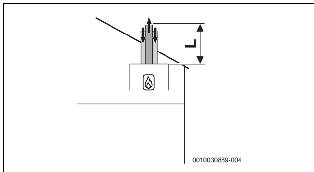
8. ábra Függőleges koncentrikus levegő-/ füstgázelvezetés a C 33x szerint
