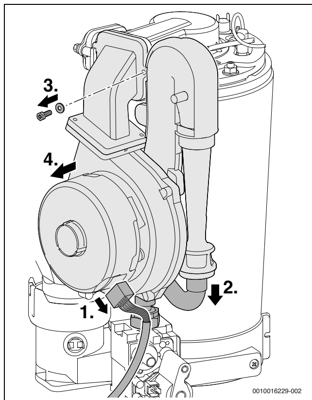
50. ábra A ventilátor és a keverőegység kiserelése
