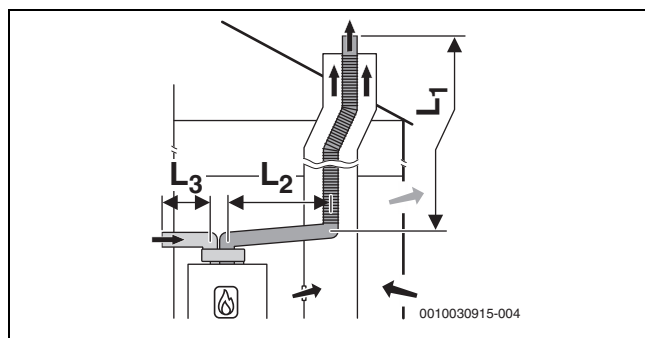
11. ábra Flexibilis fűtgázvezetés a C 53 szerint az aknában és különálló, egyfalú levegőellátó- és fűtgáz-vezetékek a felállítási helyiségben
