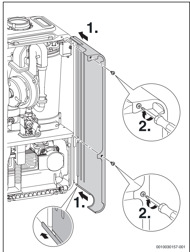
77. ábra Az oldalburkolat visszahelyezése
