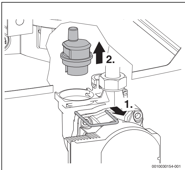
71. ábra Az automatikus légtelenítő kiszerelése
