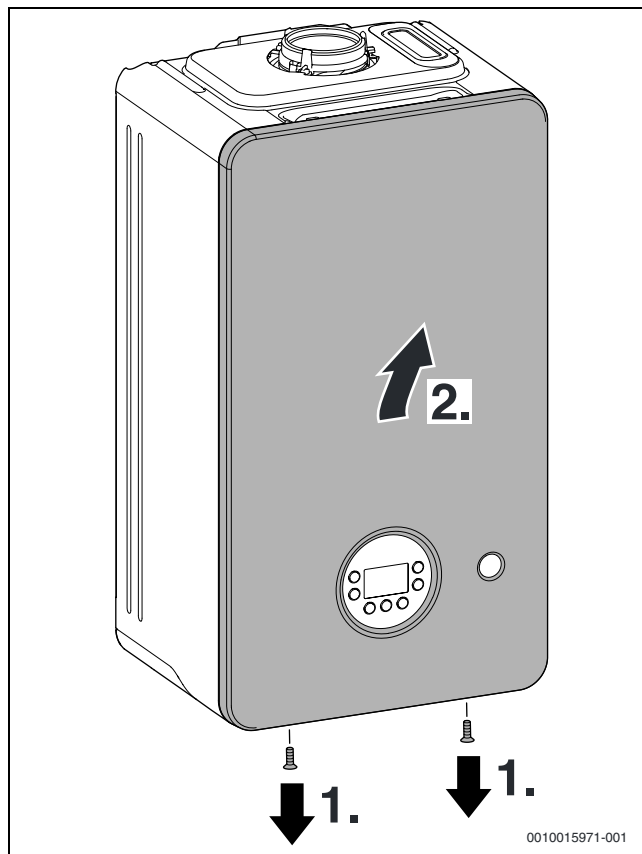
31. ábra Vegye le az előlő burkolatot
