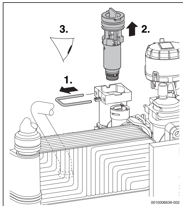
66. ábra A hidegvíz-csőben lévő szita ellenőrzése
