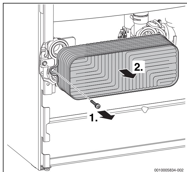
67. ábra A lemezes hőcserélő kiserelése
