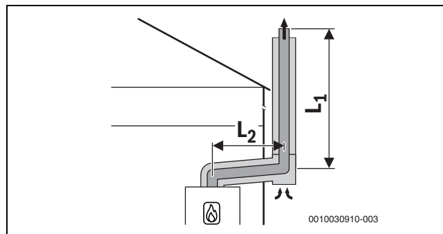
12. ábra Koncentrikus levegő-/fűtgázvezetés a C 53x szerint a külső falon
