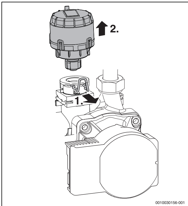
72. ábra Váltószelep motorjának kiszerelése
